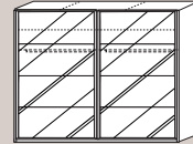
Schwebetürenschränk 53618/864 B293 x H224 x T67
